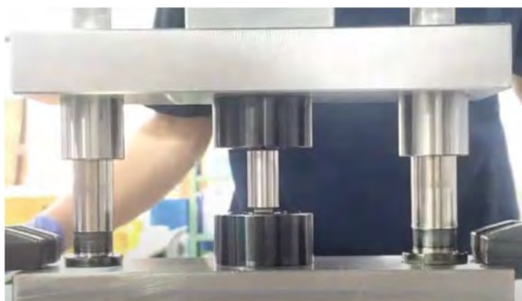
写真：カシメ接合の作業風景
